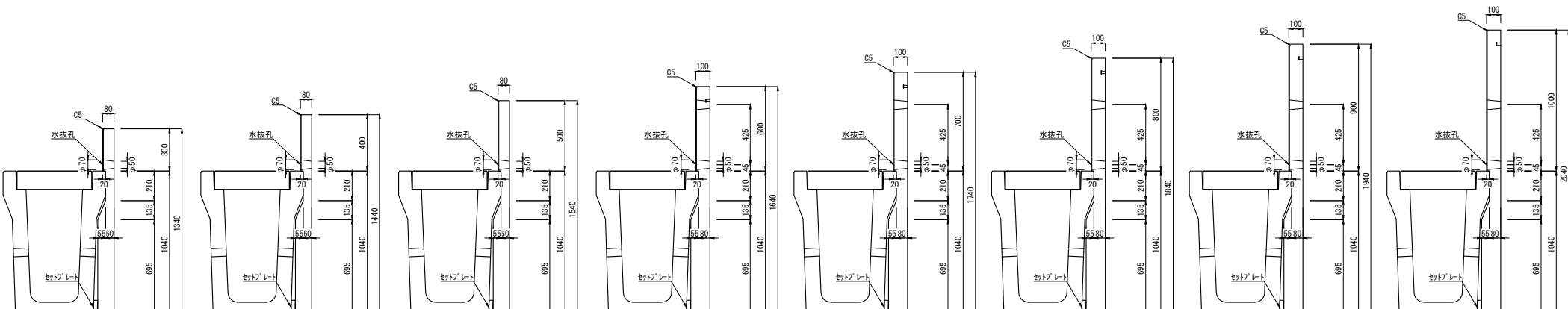
KDR400 × 800 H=300 KDR400 × 800 H=400 KDR400 × 800 H=500 KDR400 × 800 H=600 KDR400 × 800 H=700 KDR400 × 800 H=800 KDR400 × 800 H=900 KDR400 × 800 H=1000
