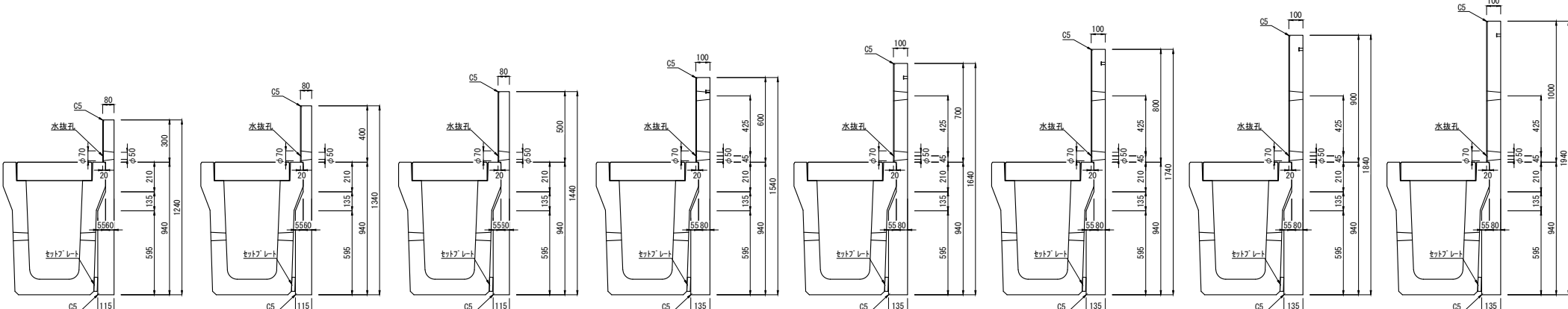
KDR400 × 700 H=300 KDR400 × 700 H=400 KDR400 × 700 H=500 KDR400 × 700 H=600 KDR400 × 700 H=700 KDR400 × 700 H=800 KDR400 × 700 H=900 KDR400 × 700 H=1000
