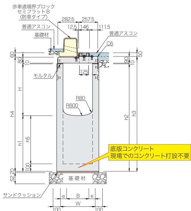
布設標準構造図(参考)
