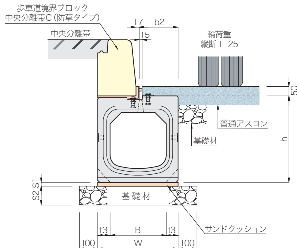
参考布設標準構造図(中央分離帯部)
