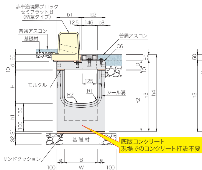
布設標準構造図(参考)
