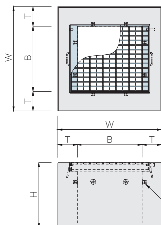
TYS 中型浸透枳500 縁塊・側塊 規格寸法表
