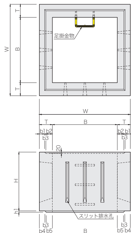
呼び名 寸法 (mm) 参考質量 (kg) W B T H h1 b1 b2 b3 b4 b5 900 1400 1000 200 900 20 80 100 20 85 95 1906 1200 1200 2520
