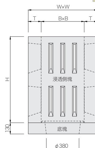
TYS 中型浸透枳500 浸透側塊 規格寸法表
