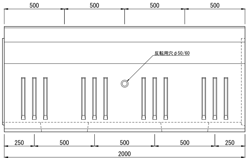
平面図
