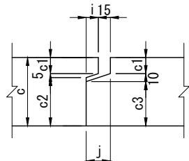
継手詳細図
