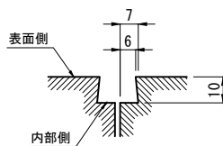
化粧目地詳細図
