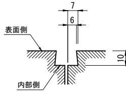
目地詳細図
